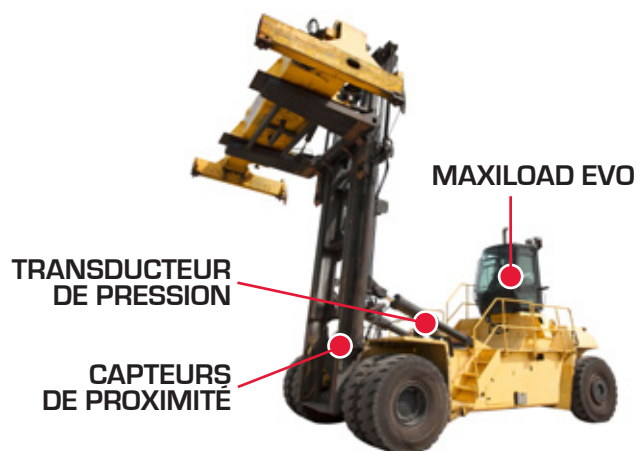
Chariot porte conteneur / prise par le dessus
